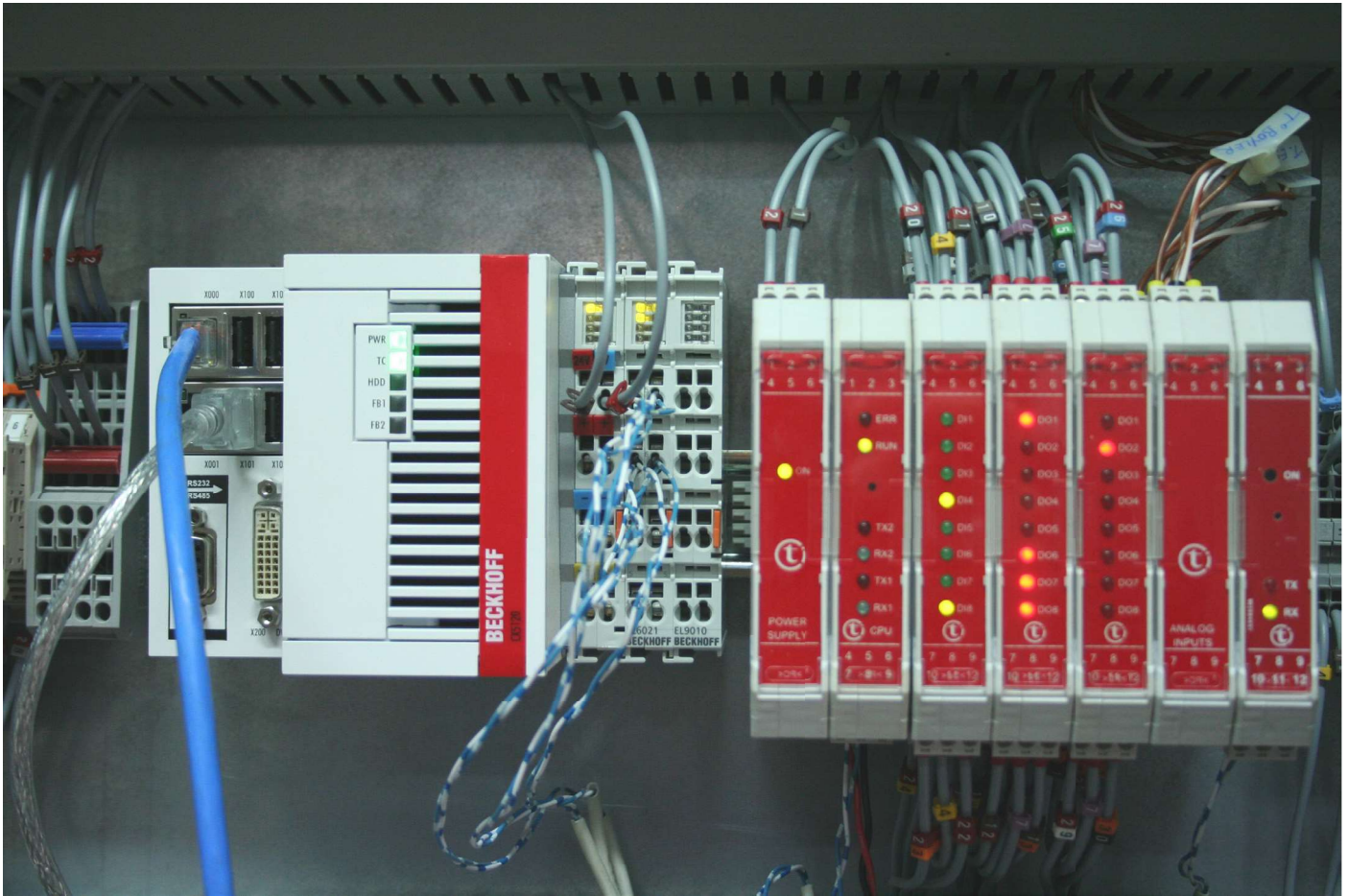
Controllore CX5120 e dispositivi di campo
